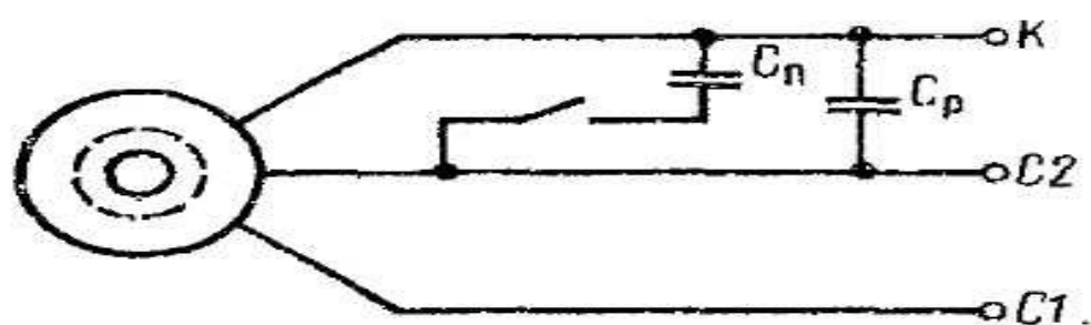
Схема включения двигателя ДС-1 ( C_n = 0,5 мкФ, 350 В; C_p = 0,5 мкФ, 350 В)
