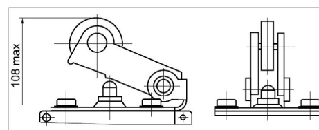
Рисунок А4 Выключатель ВПК2112
