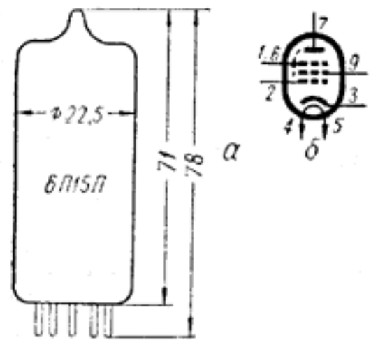
Рис. 417. Лампа 6П15П: а — основные размеры; б — схематическое изображение; 1 и 6 — третья сетка и внутривламповый экран; 2 — первая сетка; 3 — катод; 4 и 5 — подогреватель (накал); 7 — анод; 8 — свободный; 9 — вторая сетка.
