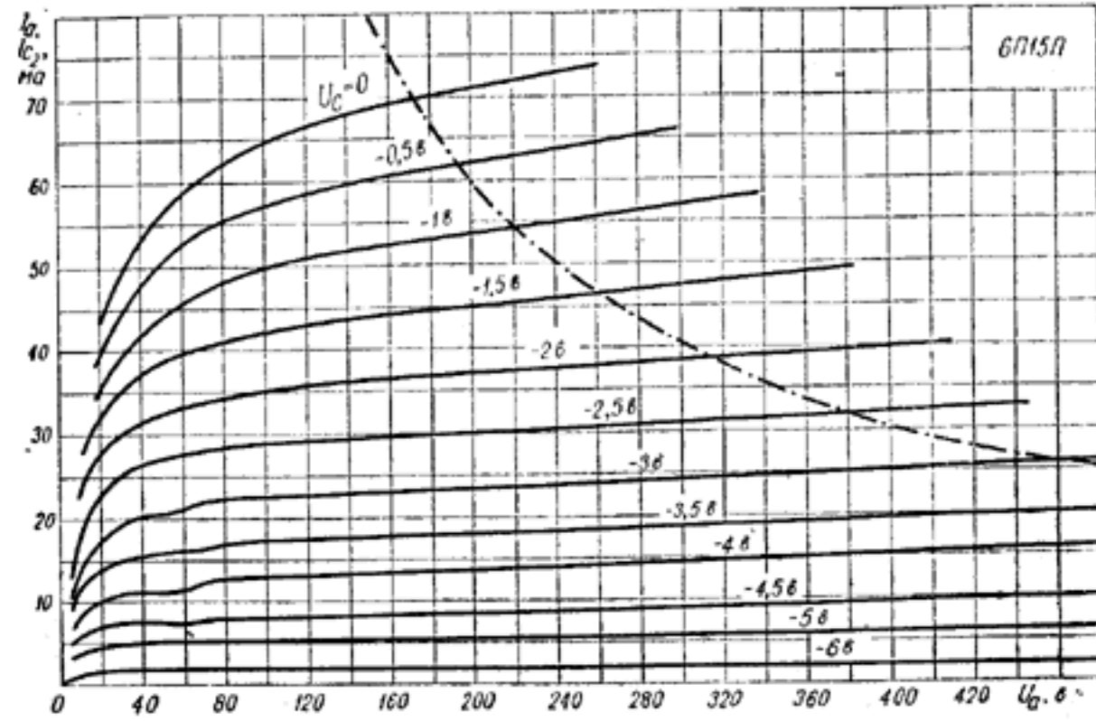
Рис. 419. Усредненные характеристики зависимости тока анода и тока второй сетки от напряжения на аноде при напряжении на второй сетке 150 в: — ток в цепи анода; - - - - - наибольшая мощность, рассеиваемая на аноде.
