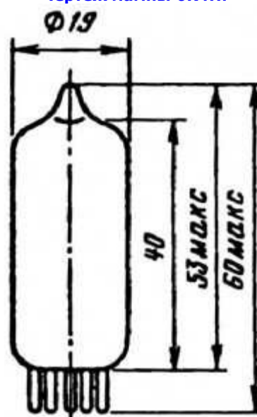
Чертёж лампы 6К4П:
