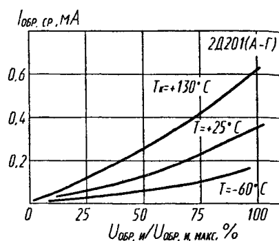
Зависимости обратного тока от напряжения
