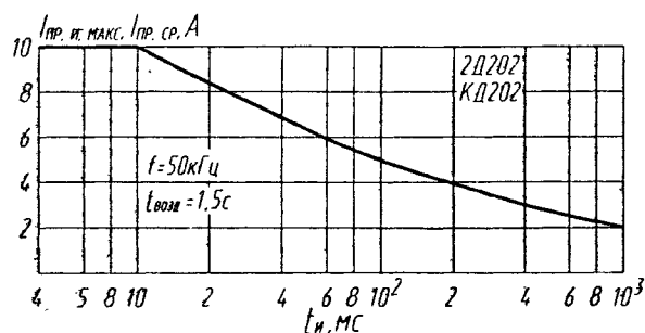
Зависимость допустимой перегрузки по импульсному прямому току от длительности импульса
