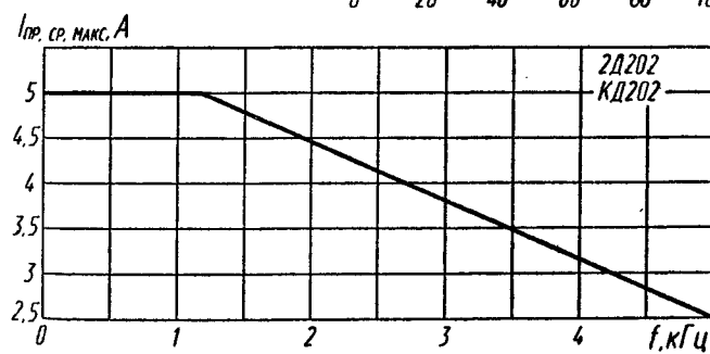
Зависимость допустимого прямого тока от частоты
