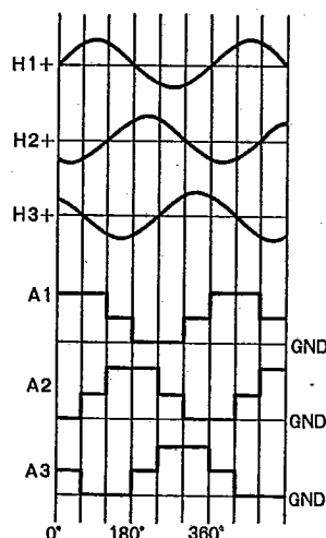
Fig.4 位相関係図
